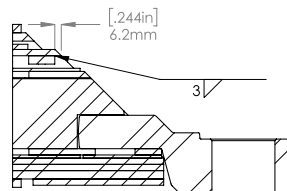
SECTION A-A SCALE 1:4
